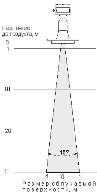
Рисунок 1 – Диаграммы направленности антенн уровнемеров
