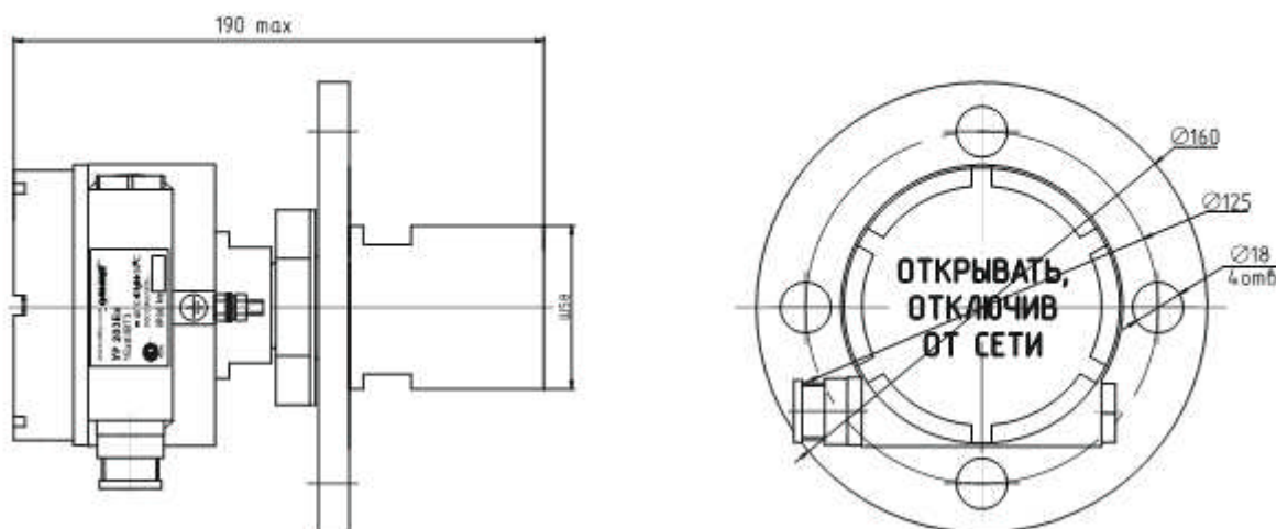
Рисунок А8 – УР203Ех с рупорно-диэлектрической антенной D = 50 мм. Установка на патрубки высотой H_n \leq 300 мм и диаметром d = 50 мм.
