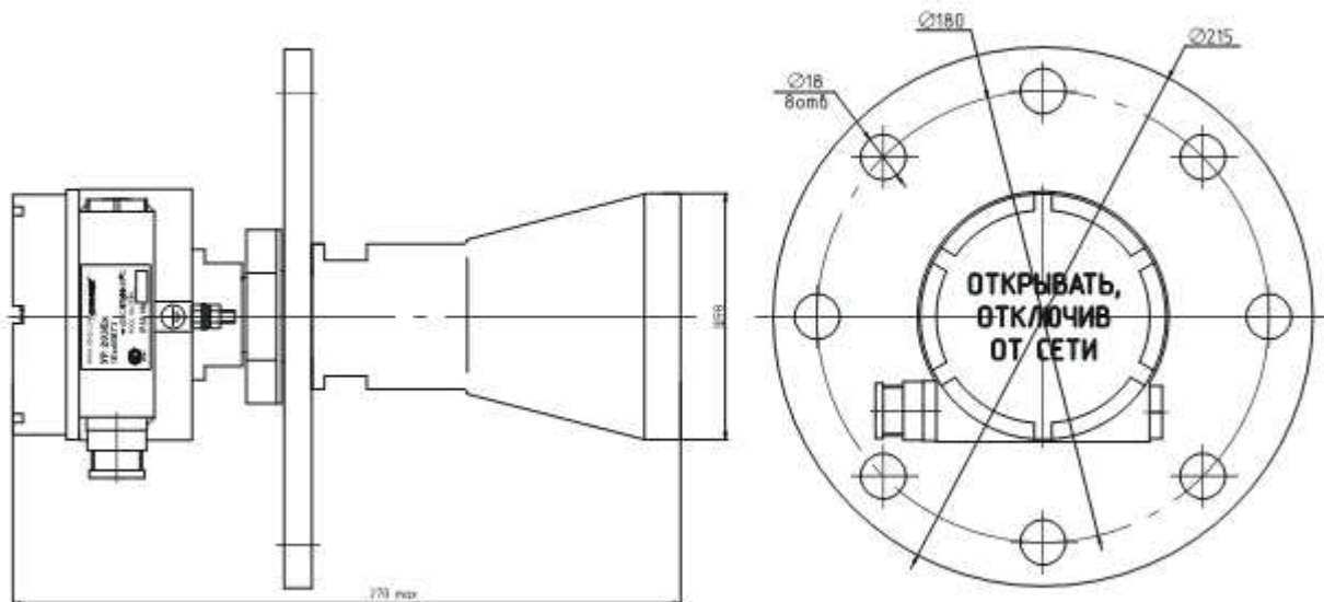
Рисунок А7 – УР203Ех с рупорно-диэлектрической антенной D = 100 мм.
