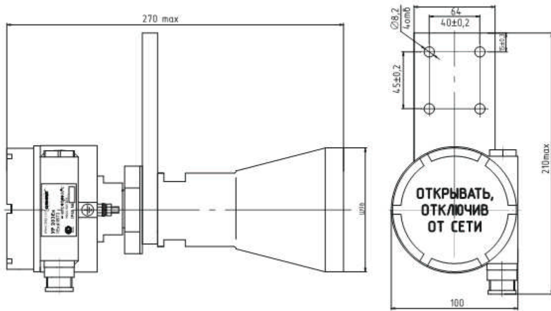
Рисунок А6 – УР203Ех
