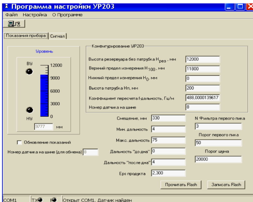
Рисунок 4 - Окно программы УР203 после установления связи с прибором
